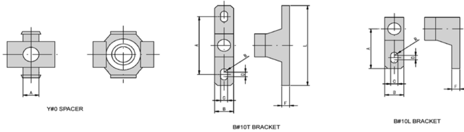
Spacer
